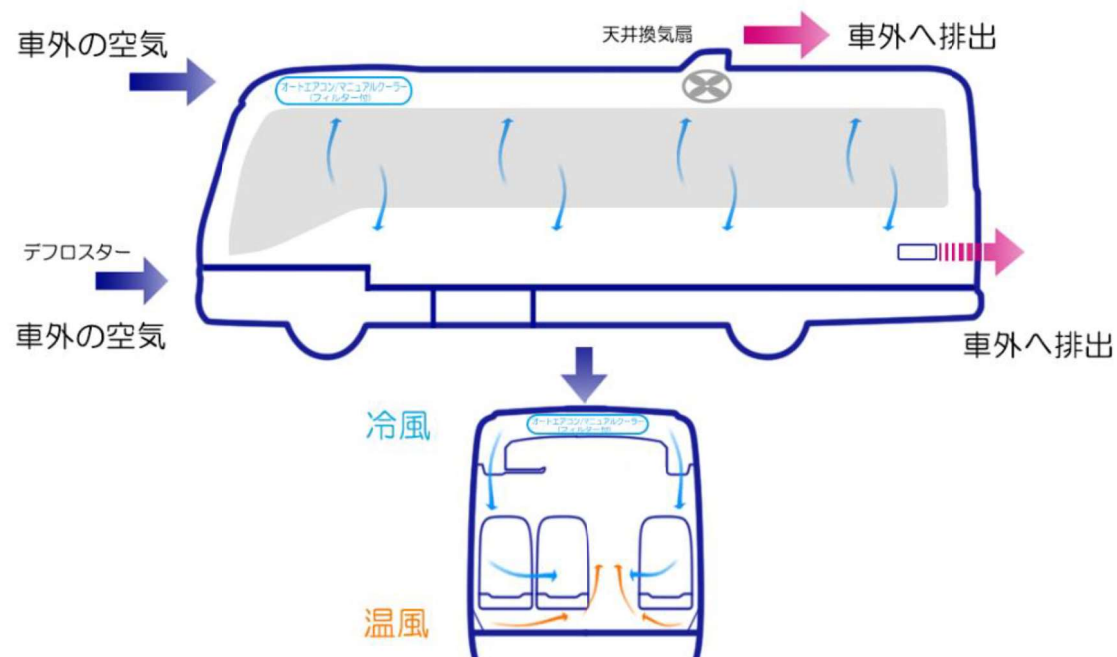
日野リエッセII 車内空調イメージ図
