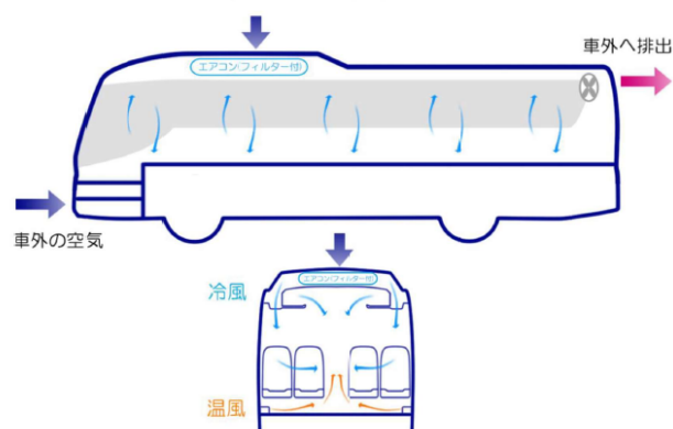
日野セレガ 車内空調イメージ図
